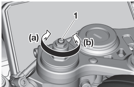
1. Regulador de la amortiguación en compresión
